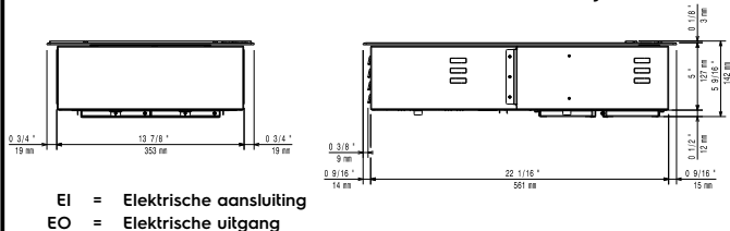
Zij aanzicht
